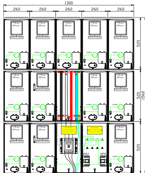
Montagem para instalação de de 05 até 12 medidores
