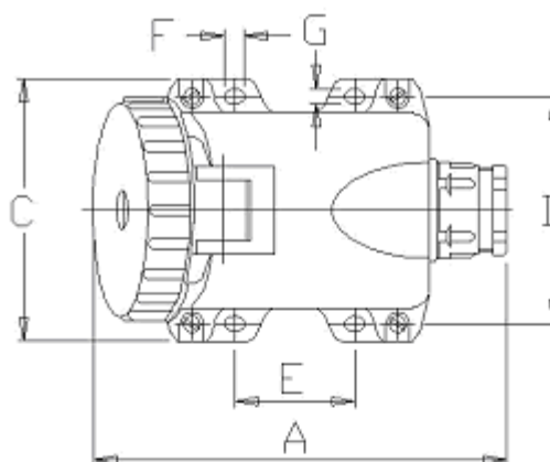
Tomada de Sobrepor - 3 POLOS
