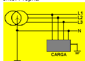
Figura 4 - Esquema TT Fonte: Própria
