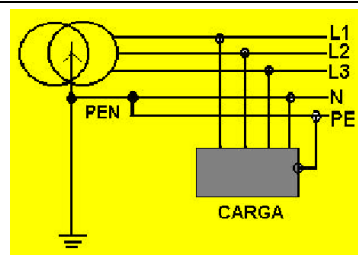
Figura 2 - Esquema TN-C-S Fonte: Própria
